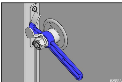
Obr. 10: Poistka pákového uzáveru s vnútorňou pákovou poistkou
